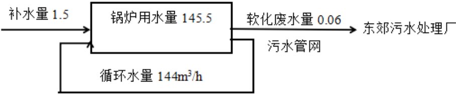
图 3 水平衡图（单位 m 3 /h）
