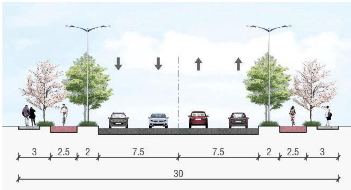
图 1 道路标准横断面图
