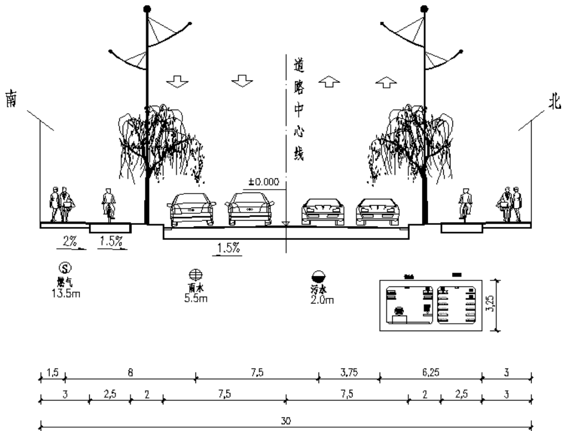
图 2 丰安路管廊与道路位置关系图
