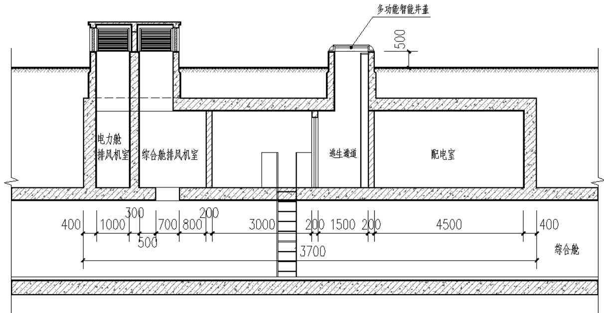
图6 通风口剖面示意图
