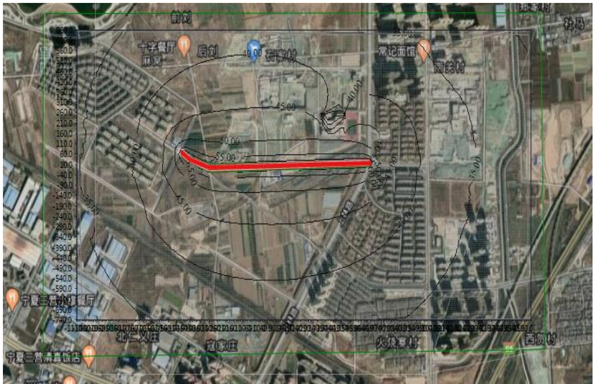
图 10 2020 年昼间噪声预测等值线图
