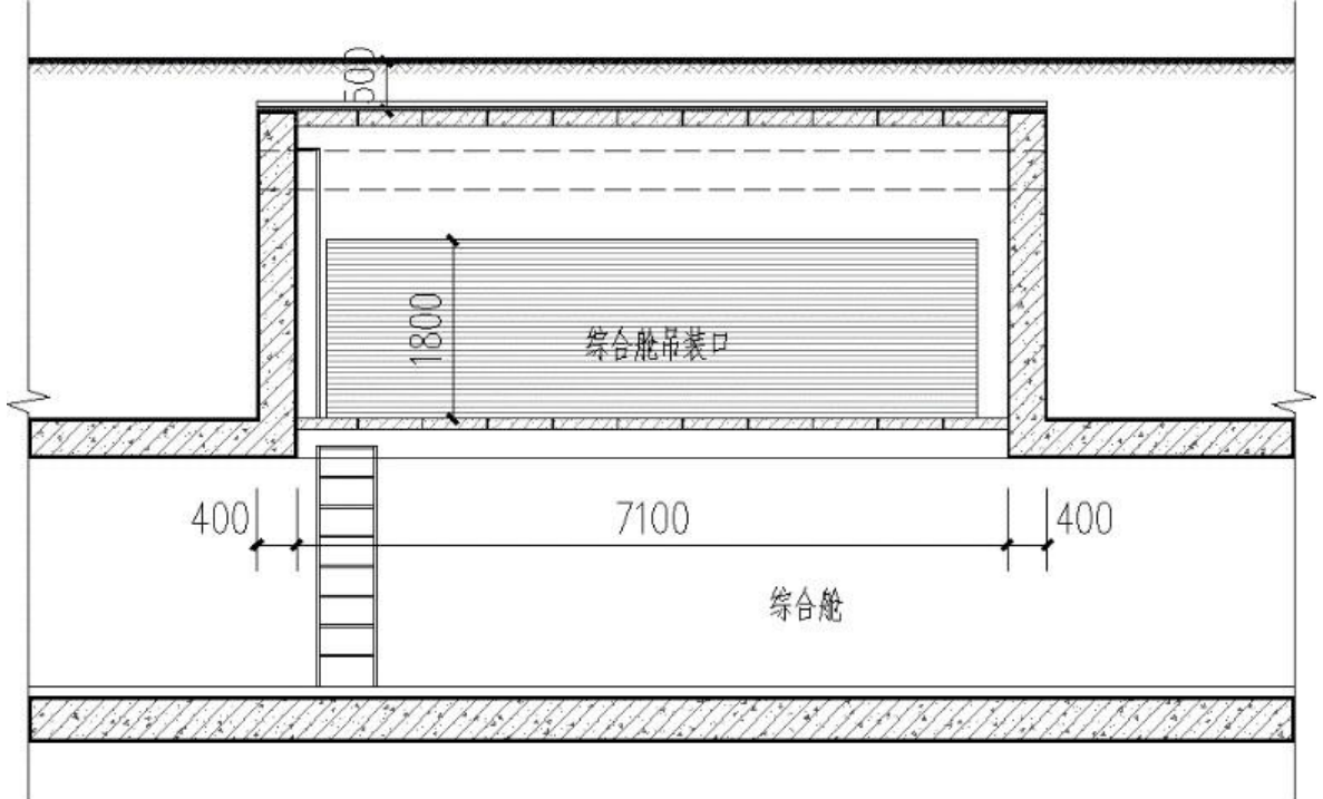
图 5 浅埋式吊装口
