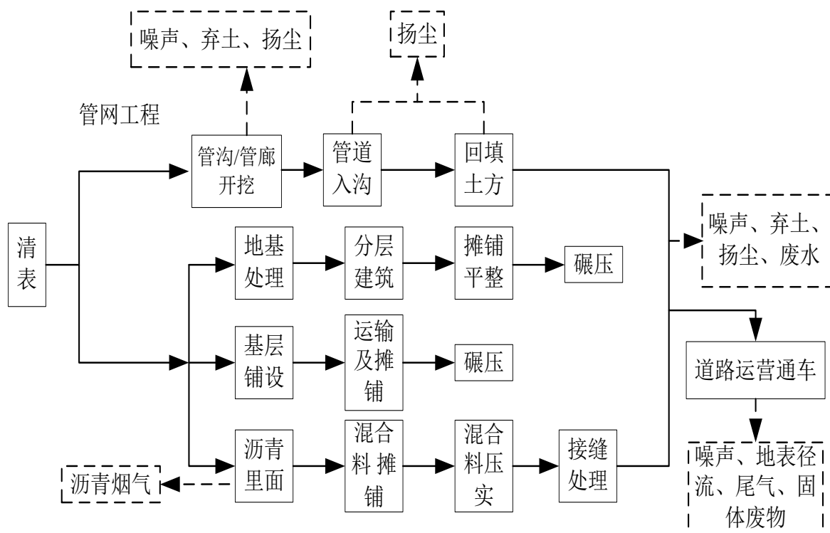
图 7 项目建设施工流程及排污节点图
