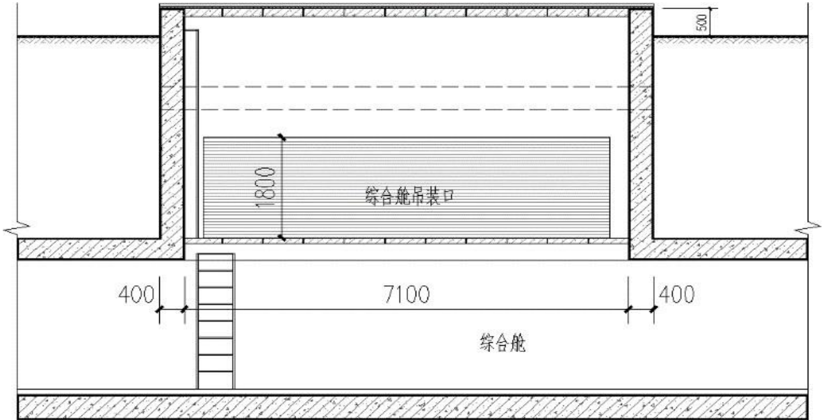
图 4 外露式吊装口
