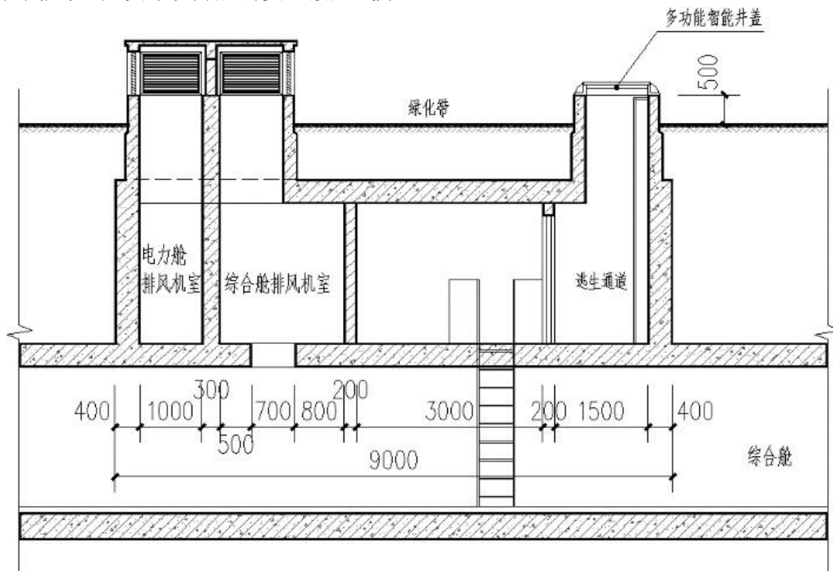
图3 逃生口剖面示意图
