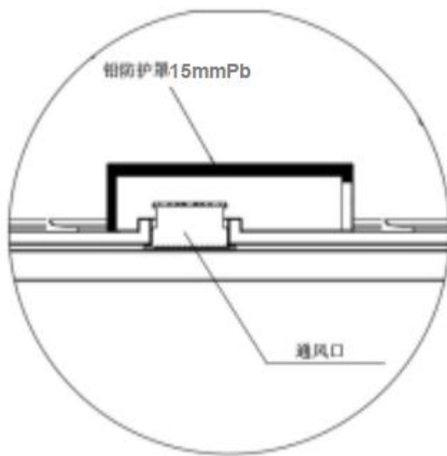
图10-6 通风口屏蔽措施示意图
