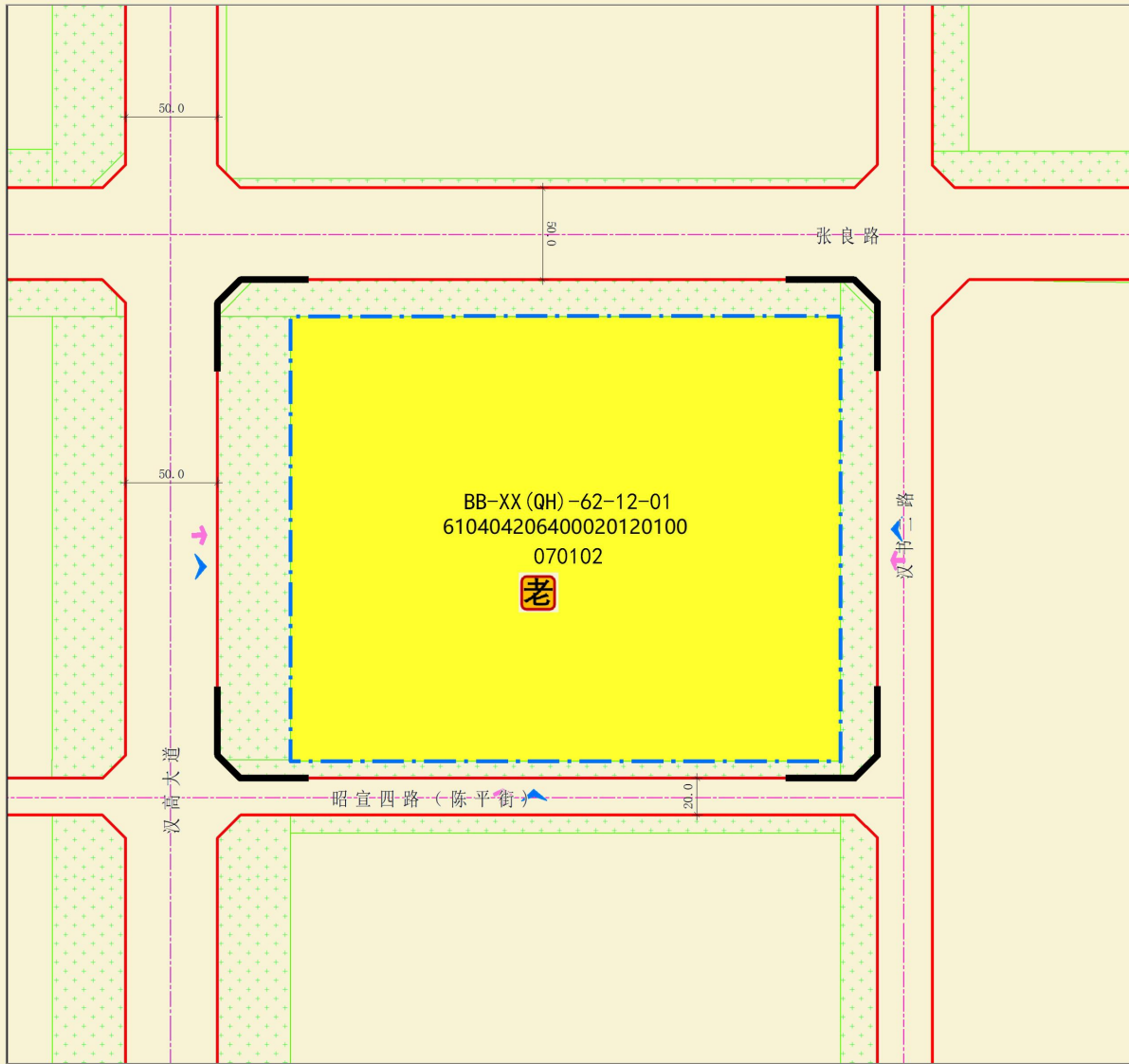
规划指标图
