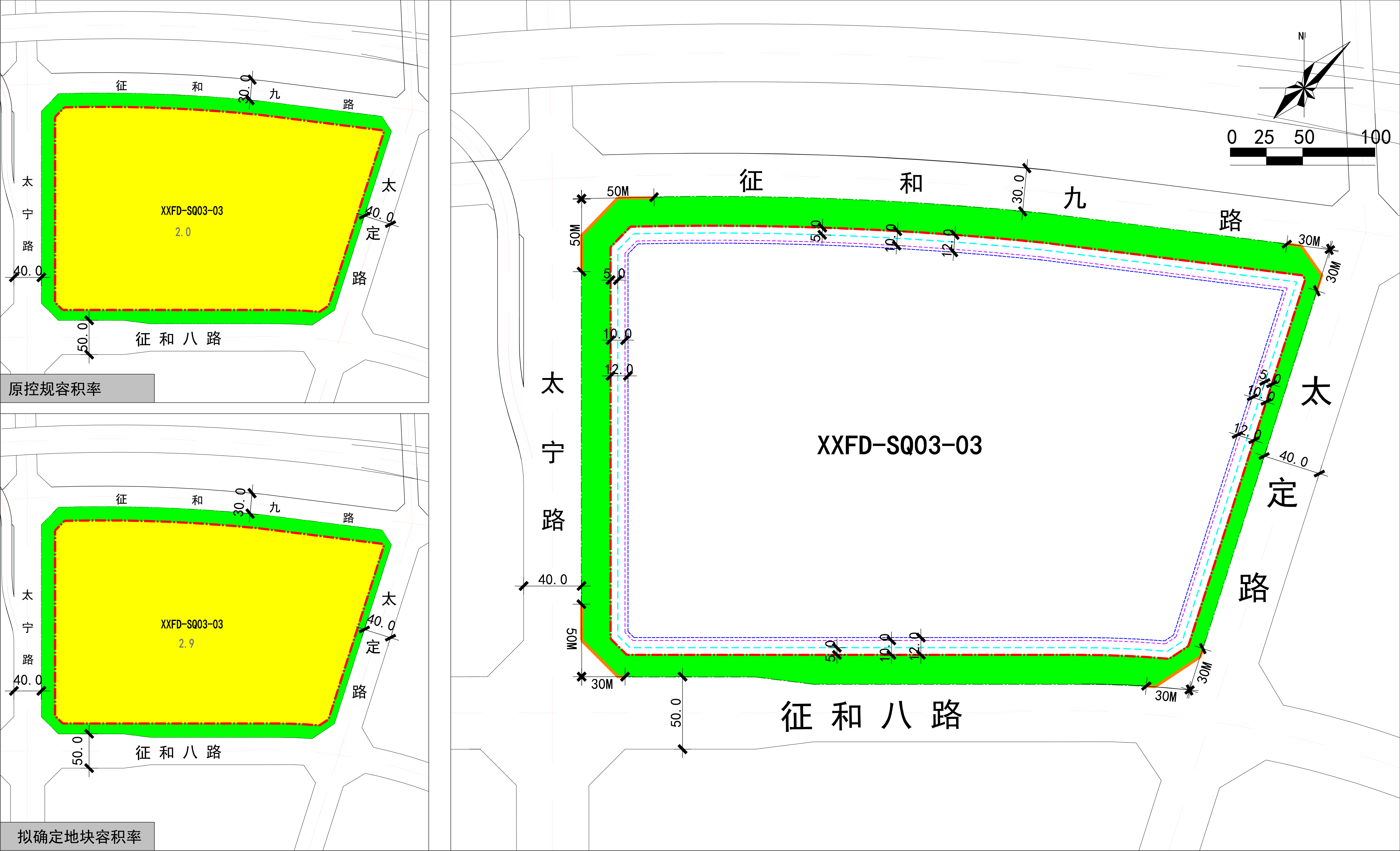
西咸新区XXFD-SQ03-03地块用地控制图
