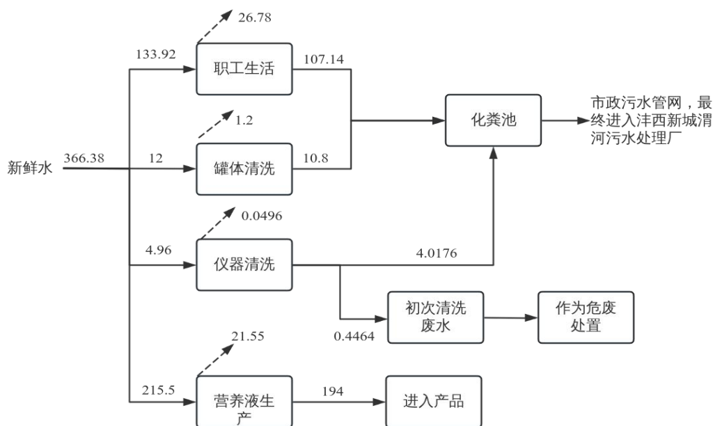
图 3-1 项目用、排水平衡图 (m 3 /a)
