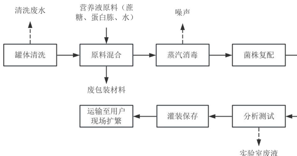
图 3-2 营运期工艺流程及产污环节图
