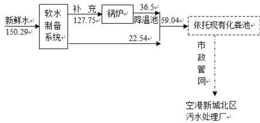
图 2-1 本项目水平衡图单位：m³/a
