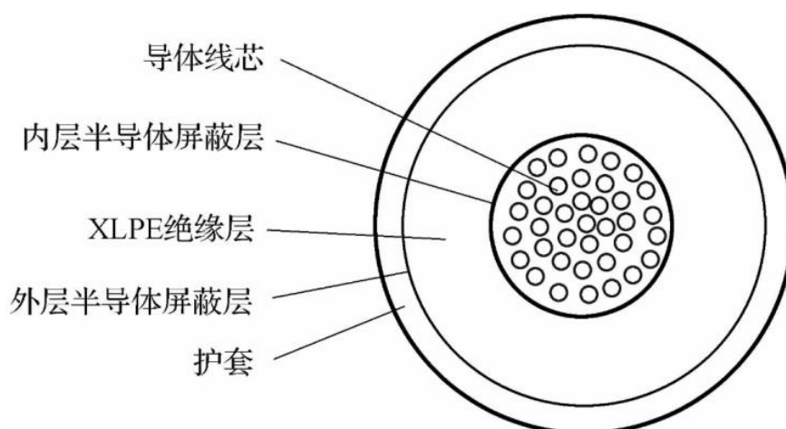
图2 电力电缆结构示意图
