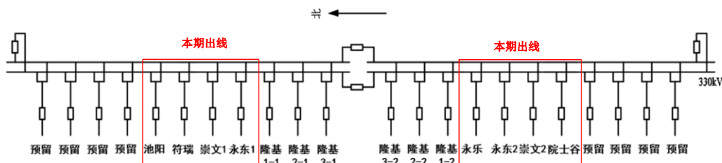
图 2-4 泾河 330kV 变电站 110kV 出线位置示意图
