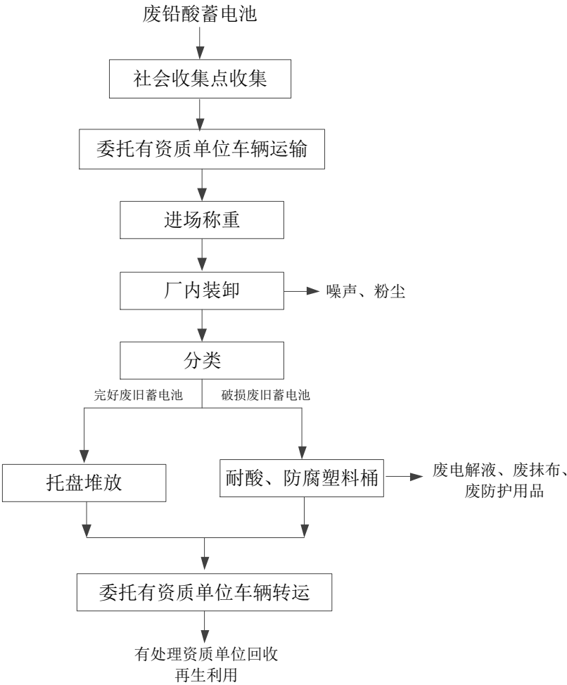
图 2 废蓄电池回收工艺流程及产污环节图
