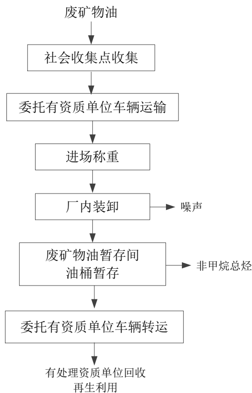
图3 废矿物油回收工艺流程及产污环节图
