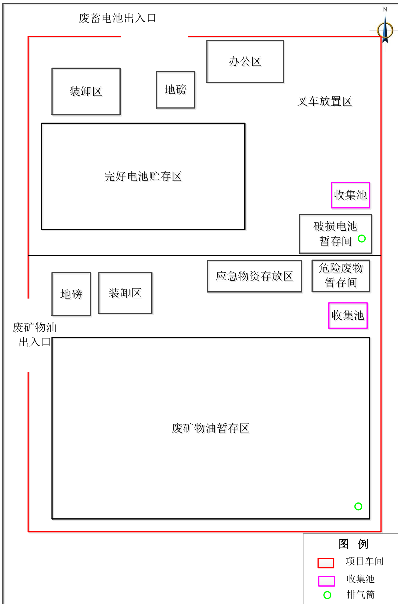
附图3 项目总平面布置图
