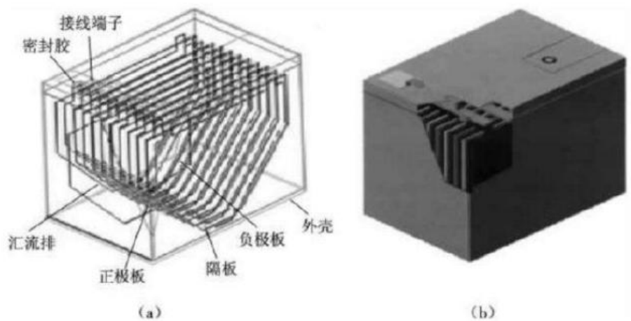
图 1 铅酸蓄电池结构示意图
