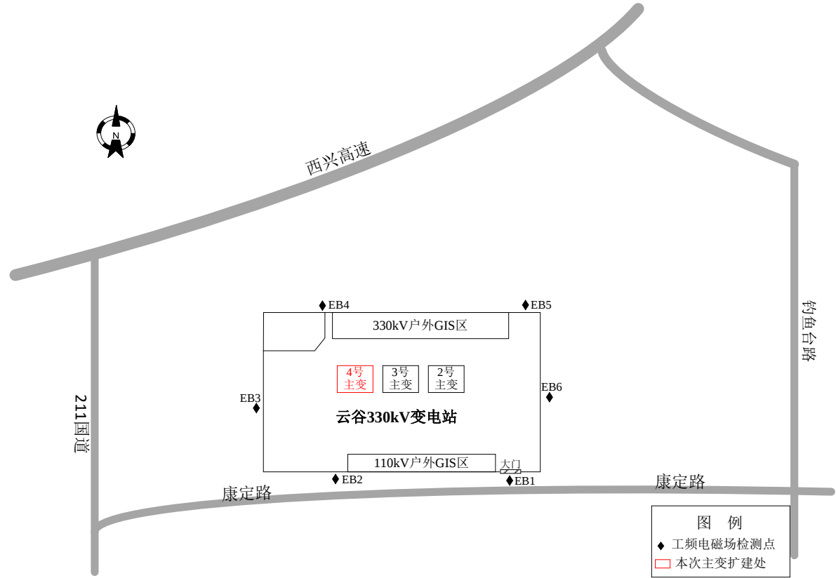
图 4.3-1 电磁环境监测点位示意图
