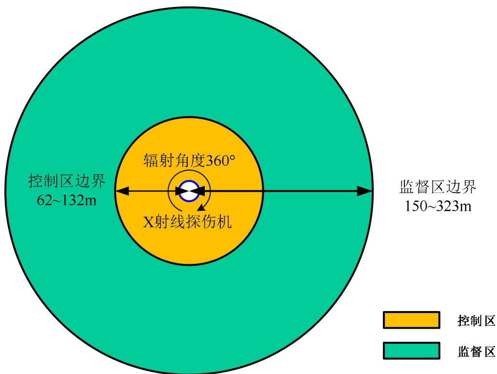
图 11-7 XXGHZ-3005 型周向 X 射线探伤机控制区和监督区范围分区示意图
