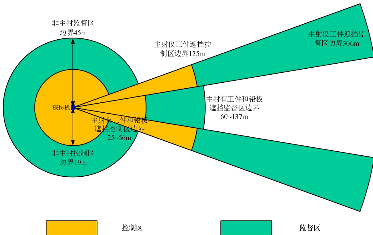
图 11-3 XXG-3005 型定向 X 射线探伤机控制区和监督区范围分区示意图
