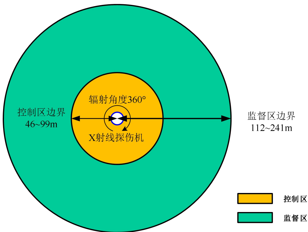
图 11-5 XXGHZ-2005 型周向 X 射线探伤机控制区和监督区范围分区示意图
