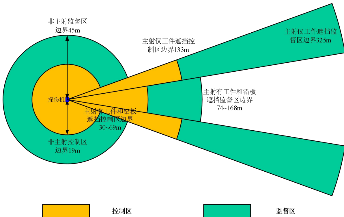
图 11-4 XXG-3505 型定向 X 射线探伤机控制区和监督区范围分区示意图
