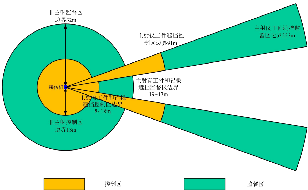
图 11-1 XXG-2005 型定向 X 射线探伤机控制区和监督区范围分区示意图
