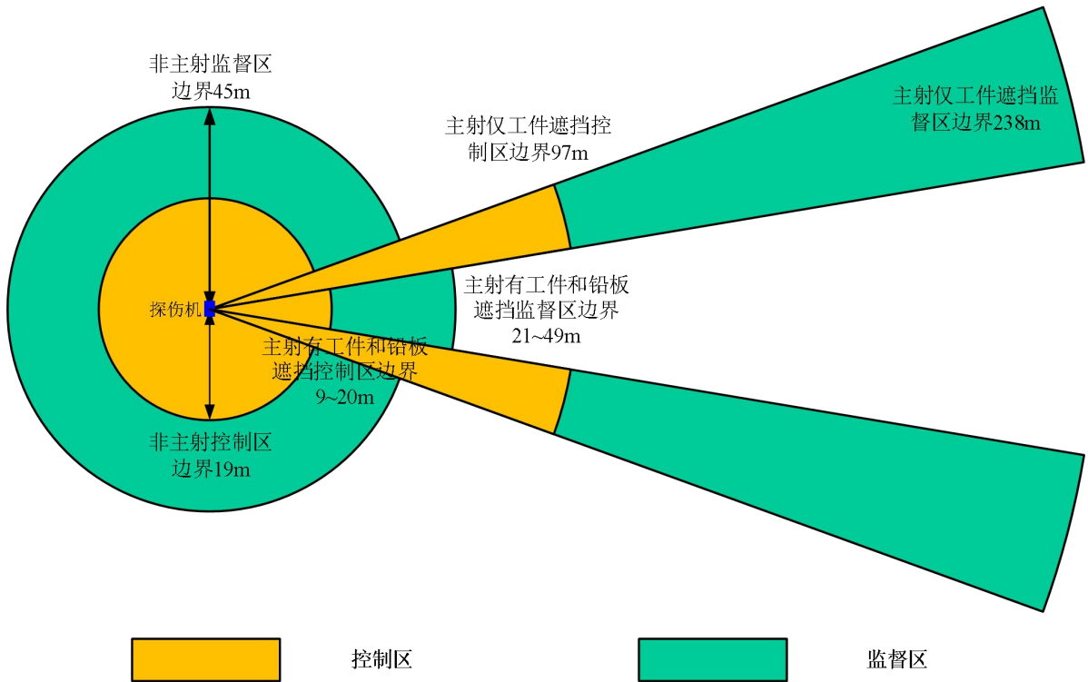
图 11-2 XXG-2505 型定向 X 射线探伤机控制区和监督区范围分区示意图
