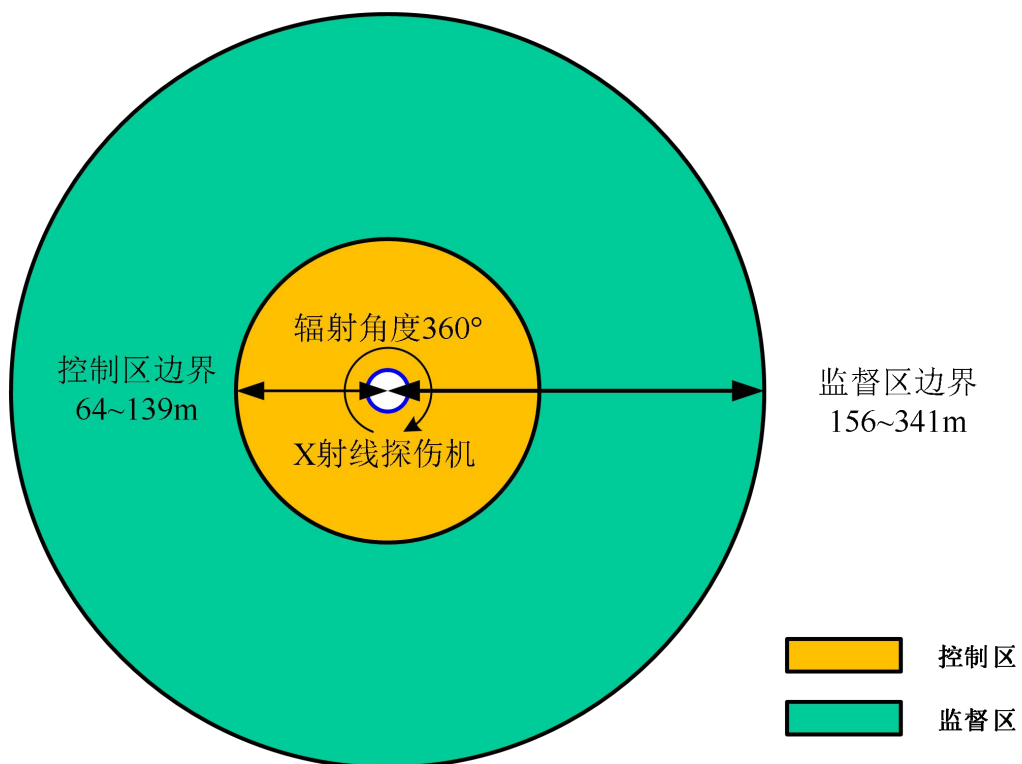
图 11-8 XXGHZ-3505 型周向 X 射线探伤机控制区和监督区范围分区示意图
