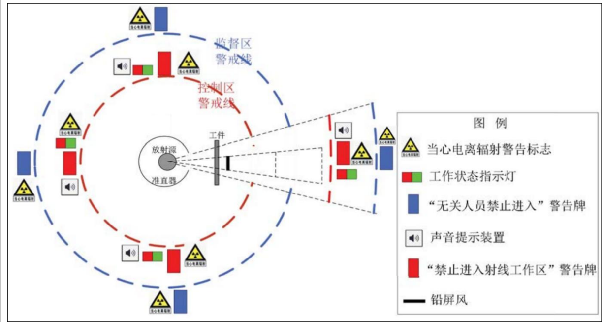
图 10-3 移动探伤现场辐射安全设施布置示意图
