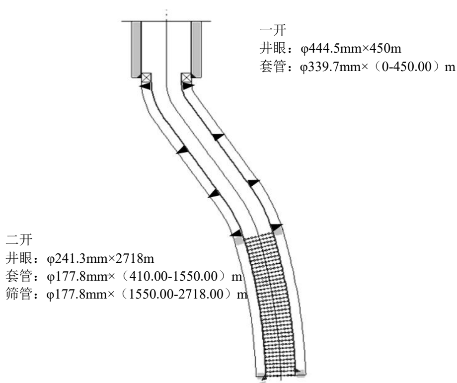
图 2-5 浅井定向井井身结构设计示意图
