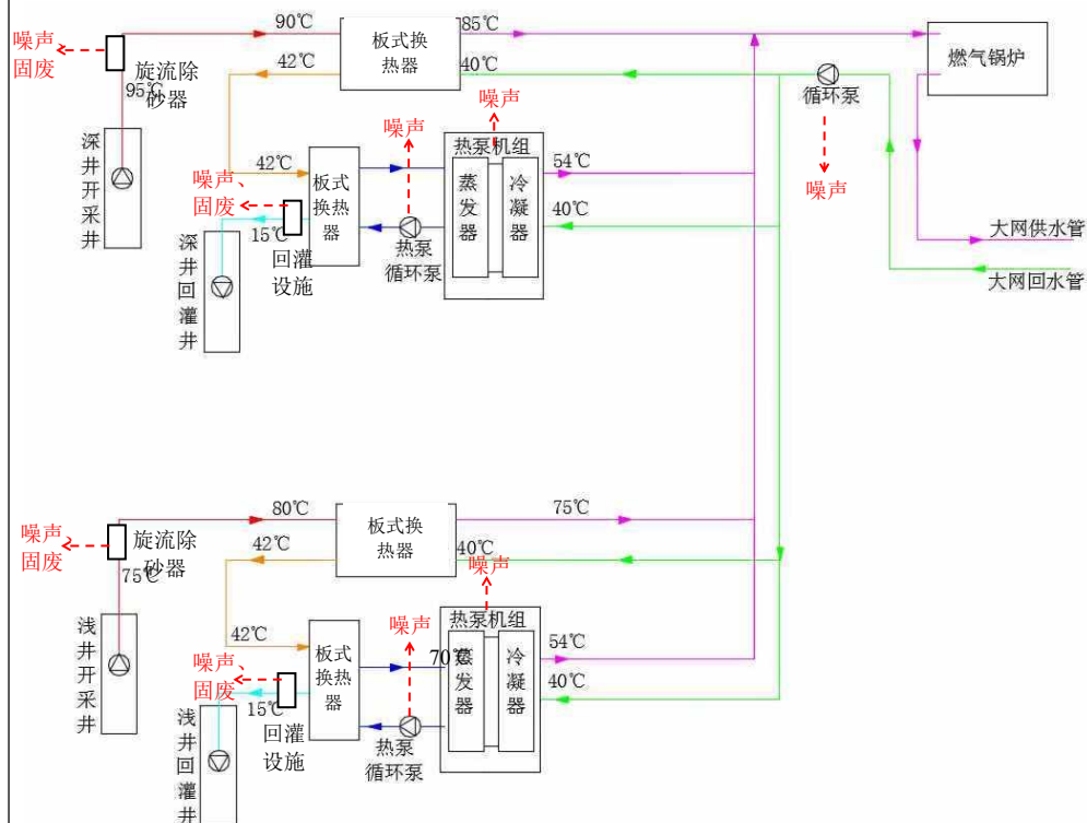
图 2-2 项目运营期工艺流程及产污环节图
