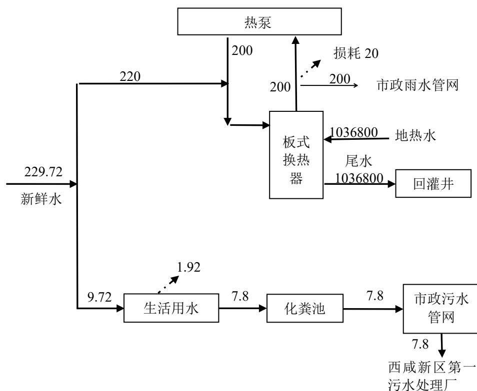
图 4-1 采暖季生产用水水量平衡图 单位：m 3 /a
