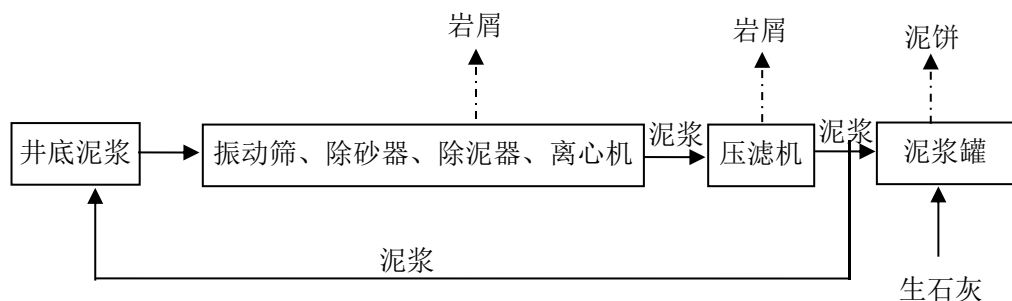
图 2-4 泥浆循环、处置工艺流程及产污环节图
