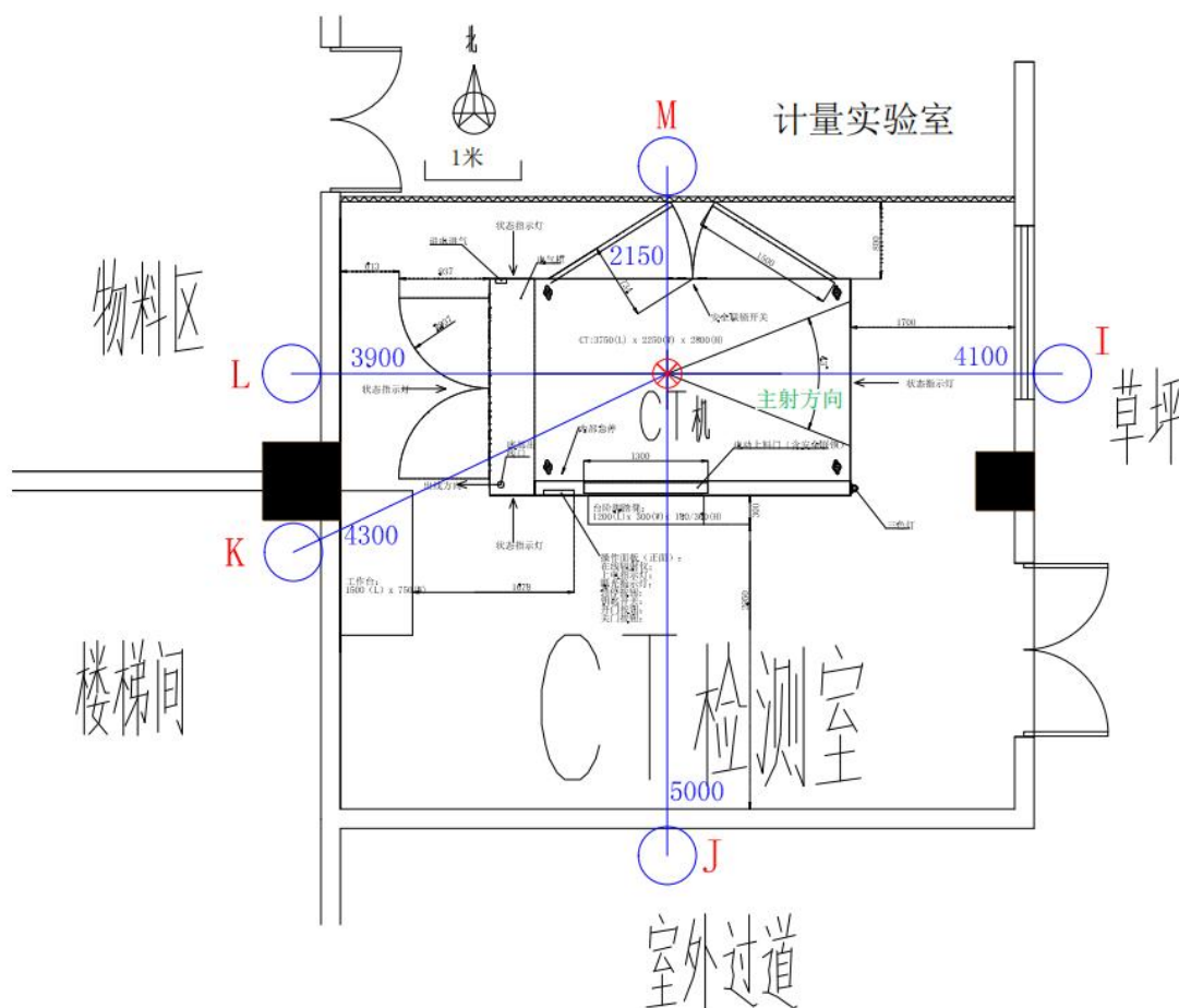
图11-3 拟建工业CT检测室外关注点示意图
