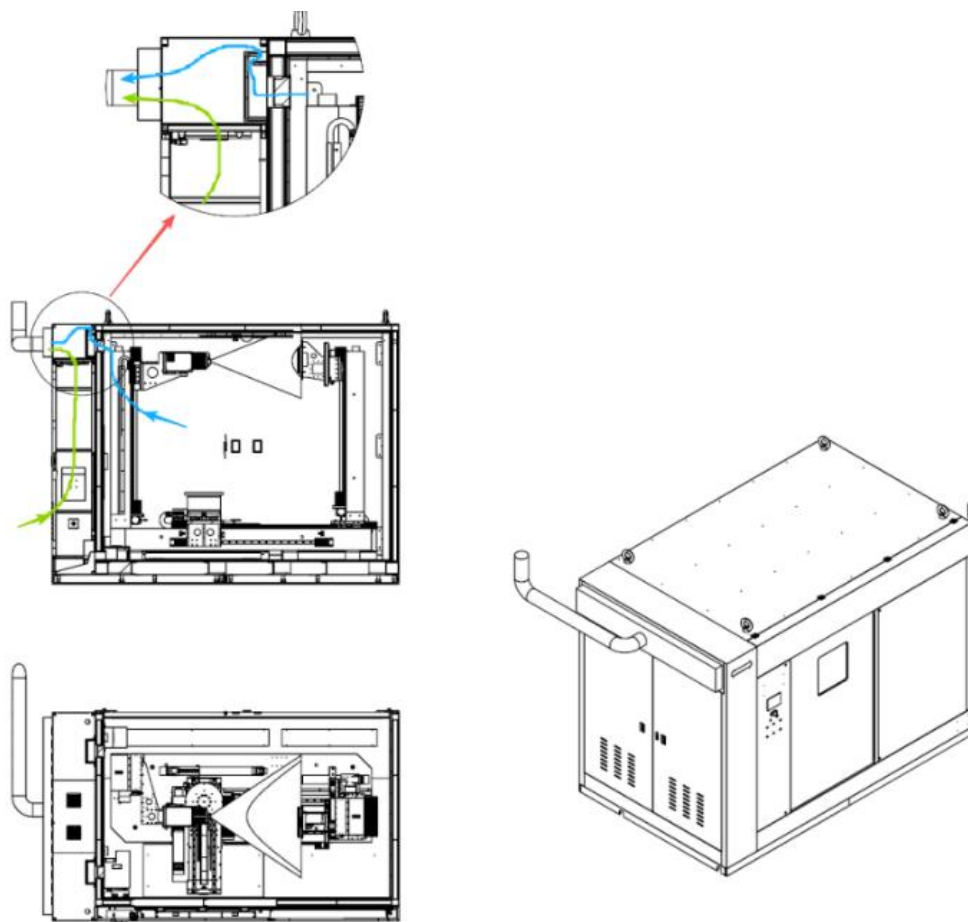
图 10-5 铅房废气排放管道设计图
