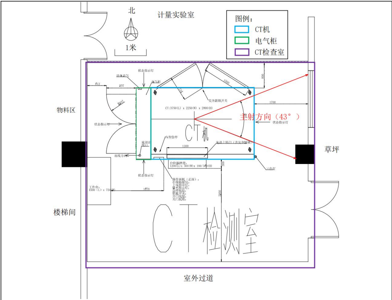
图 1-6 CT 检测室平面布置图
