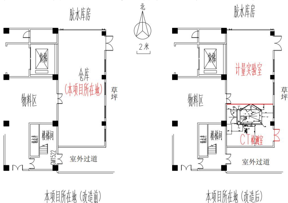
CT 检测室依托 9#厂房东北侧仓库建设，现为闲置状态，该仓库拟隔断出两间房间，南侧为 CT 检测室，北侧为计量实验室，仓库改造前与改造后情况详见平面图 1-4。
