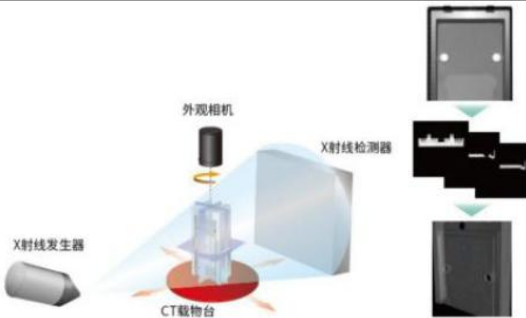
图 9-4 工业 CT 检测原理图
