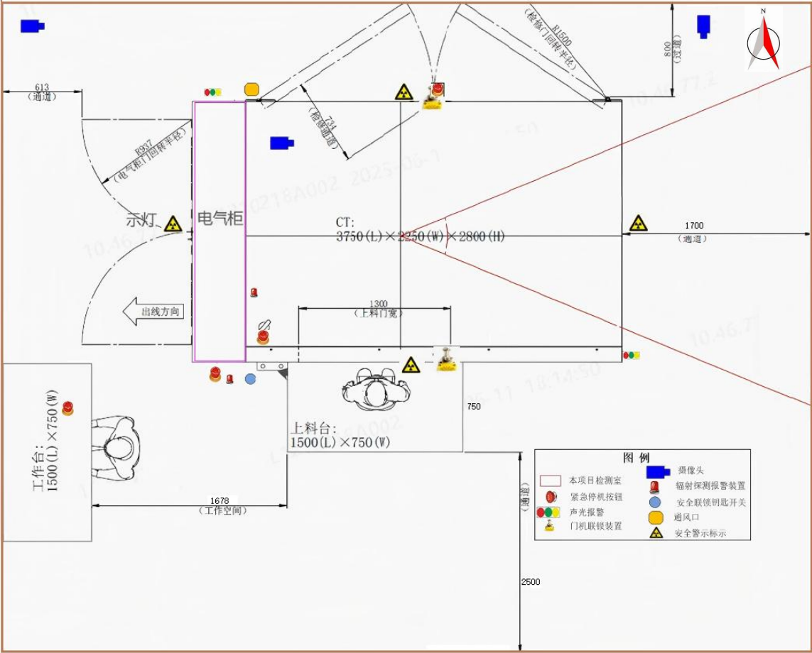
图 10-4 辐射安全与防护设施位置示意图
